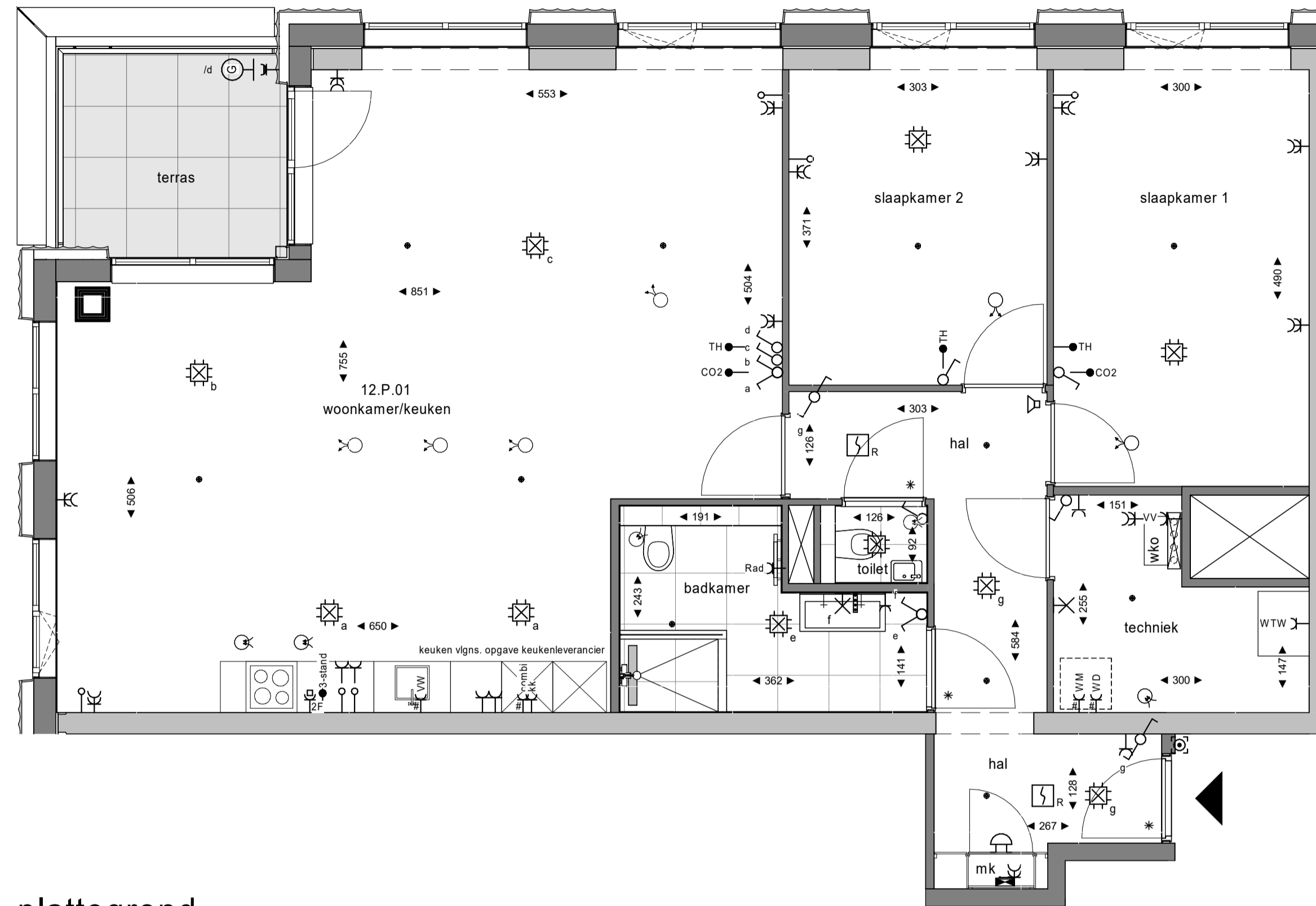
plattegrond 1 : 50 12e verdieping
