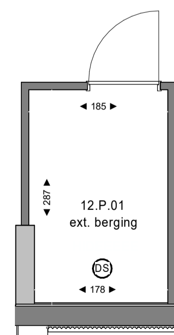
plattegrond berging 1 : 50 4e verdieping
